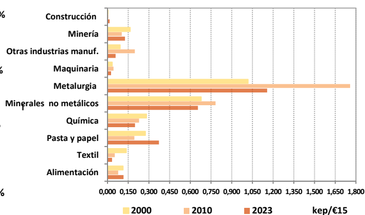
Intensidad energética de la industria por ramas, 2000-2023 (8)
