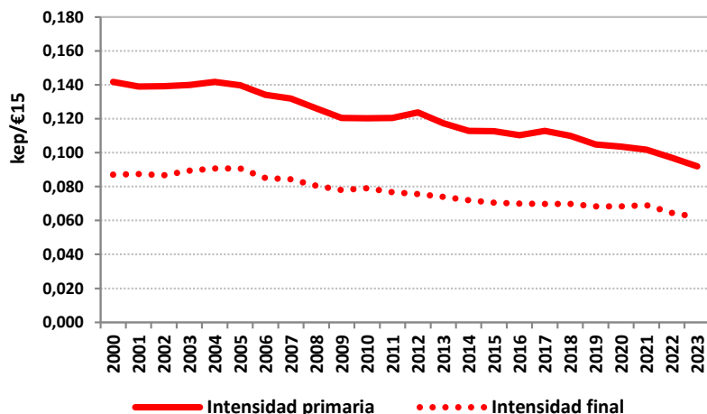
Evolución de las intensidades de energía primaria y final, 2000-2023 (7)
