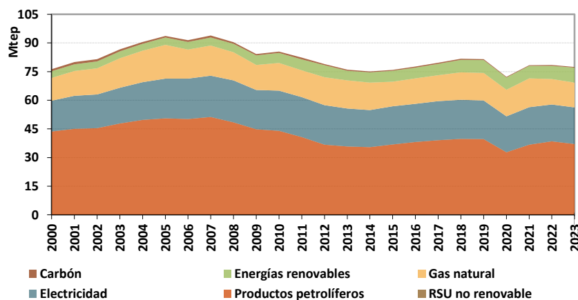
Evolución del consumo de energía final por fuentes energéticas, 2000-2023 (2)
