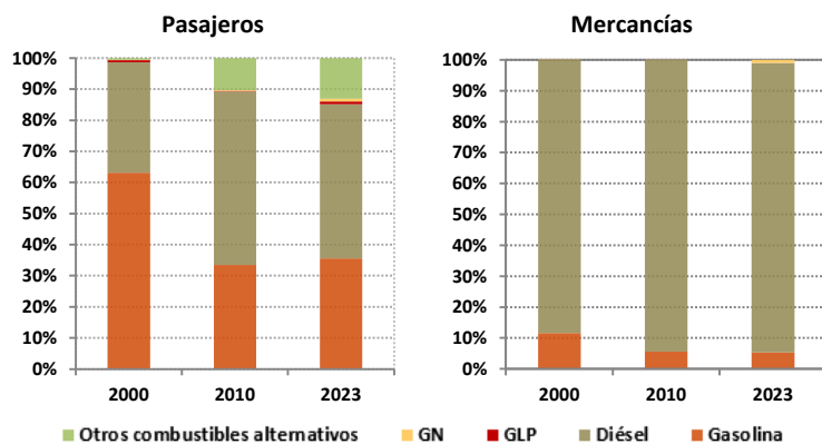
Estructura del consumo energético del transporte en carretera por fuentes energéticas, 2000-2023 (13)(15)
