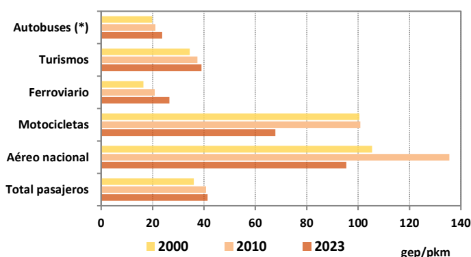
Consumo unitario del transporte de pasajeros por tipos de vehículos, 2000-2023 (13)(18)
