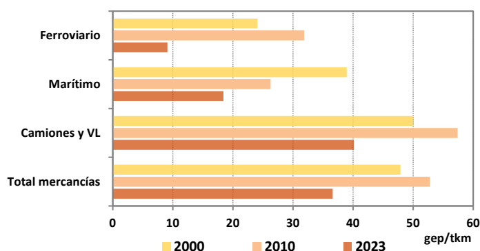
Consumo unitario del transporte de mercancías por tipos de vehículos, 2000-2023 (13)(14)(18)
