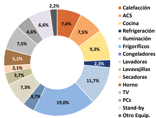
Estructura del consumo eléctrico por tipo de equipamiento 2023 (21)
