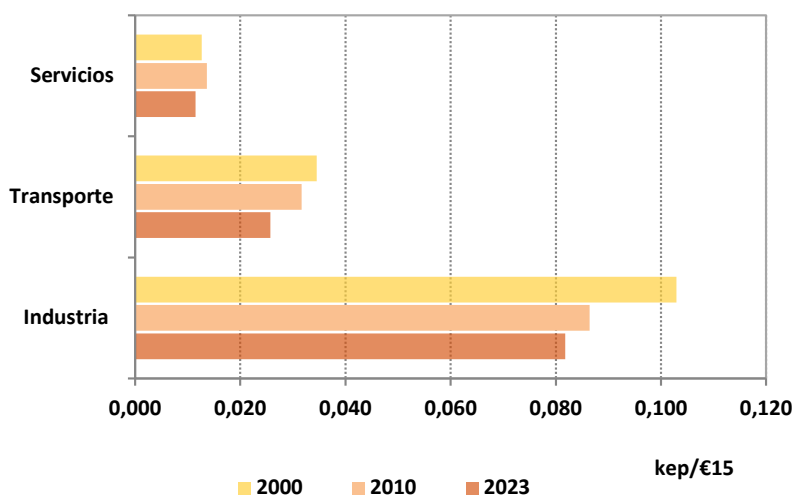
Intensidad energética de los principales sectores económicos, 2000-2023 (8)
