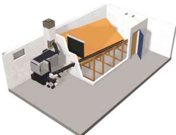
Figura 24: Almacenamiento con dos lados inclinados
