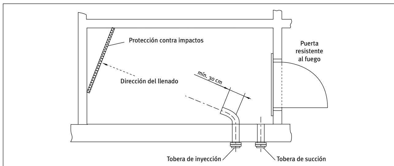
Figura 41: Silo con tobera en diagonal para un mejor llenado del espacio de almacenamiento
