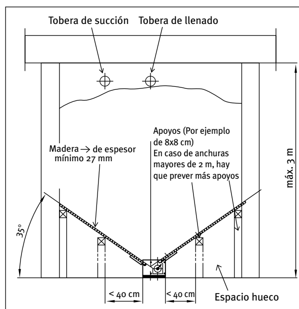
Figura 36: Disposición de las toberas en el silo
