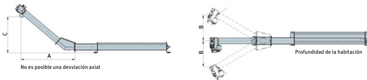
Figura 46: Disposiciones posibles del tornillo sinfín en codo
