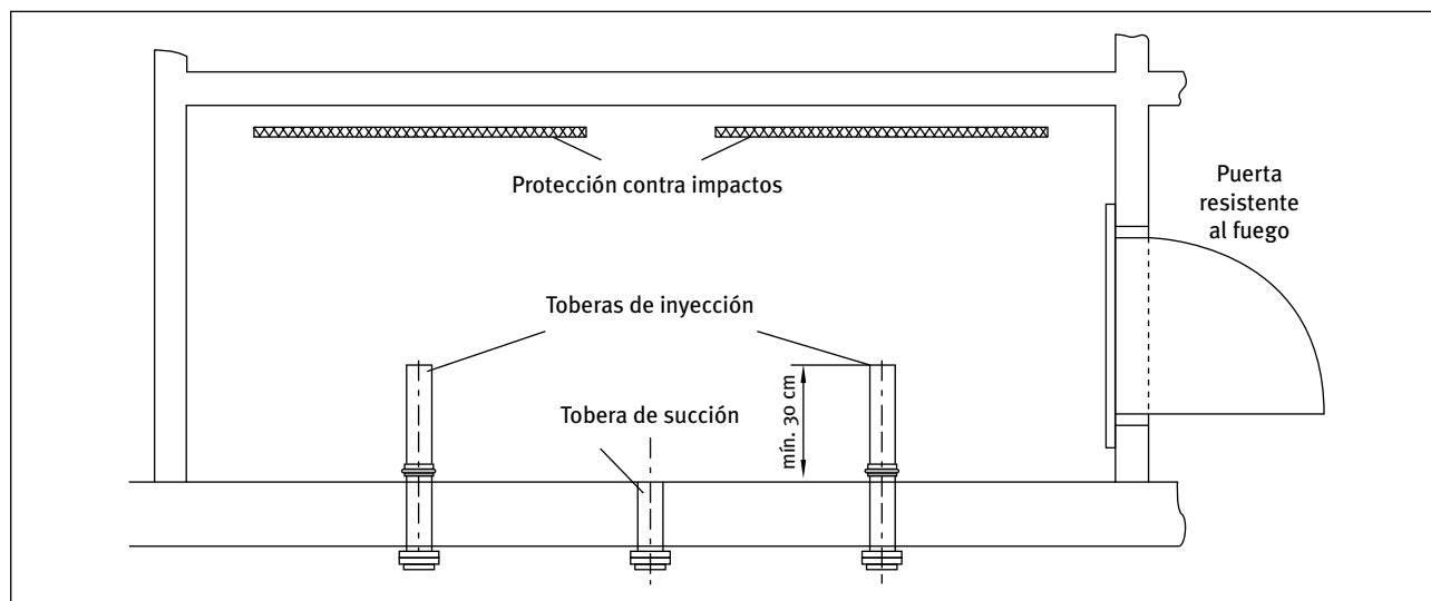
Figura 40: Silo con disposición de las toberas a lo ancho Fuente: Norma austriaca Ö NORM M7137
