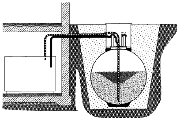
Figura 19: Depósito subterráneo para pélets Fuente: Norma austriaca ÖNORM M7137
