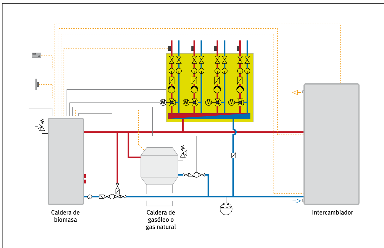
Figura 58: Caldera de biomasa con caldera convencional
