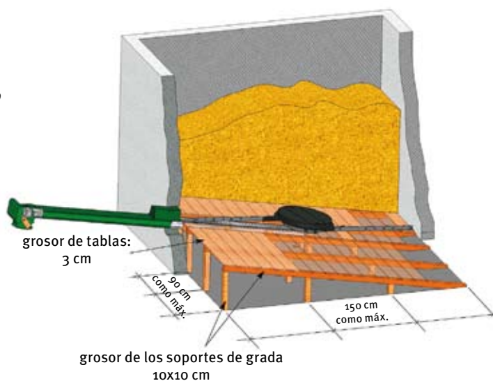
Figura 30: Almacenamiento con suelo inclinado
