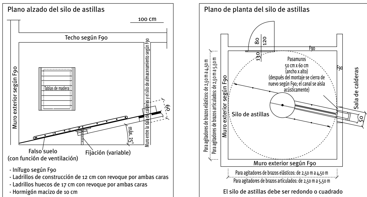
Figura 31: Silo de almacenamiento con un lado inclinado y agitador
