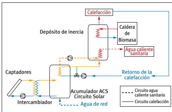
Figura 57: Sistema de distribución de calefacción y ACS centralizada
